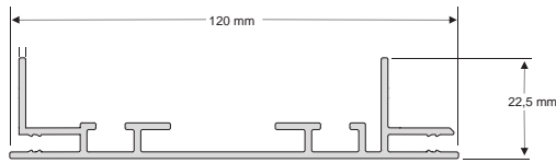
Profilquerschnitt Intex Lux
