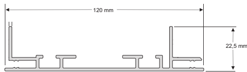
Profilquerschnitt Intex Lux Intex Lux profile
